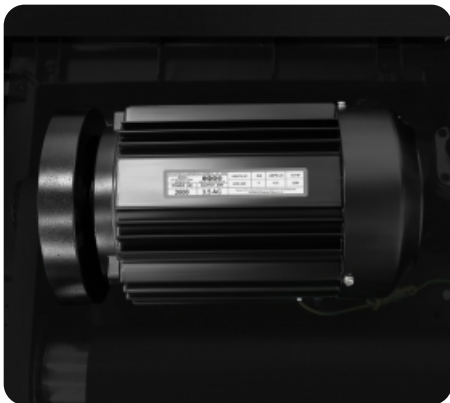
Двигатель от японского производителя Fuji Electric мощностью 3.5 л.с. (переменный ток AC)
